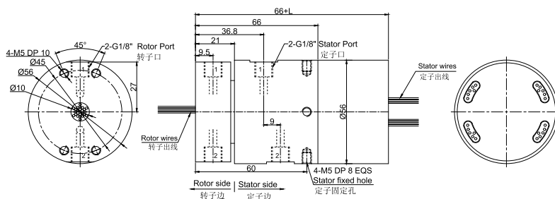
MK21+MT1256(30路及以上)尺寸图, 2进2出G1/8牙 + 信号 (5A) /10A
