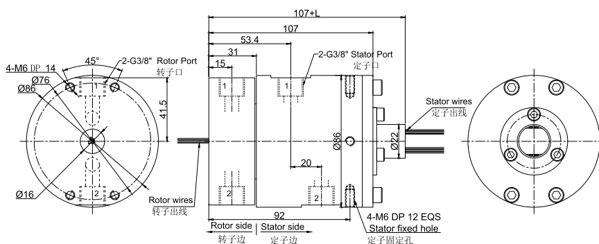
MK23S-S12(S18,S24,S36) 尺寸图 2进2出G3/8"牙+12~36路信号(2A)
